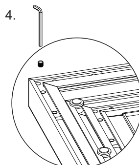
DETALHE FRAME MONTADA
