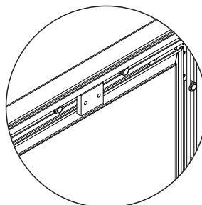
DETALHE FRAME SUPORTE PARA FIXAR NA PAREDE
